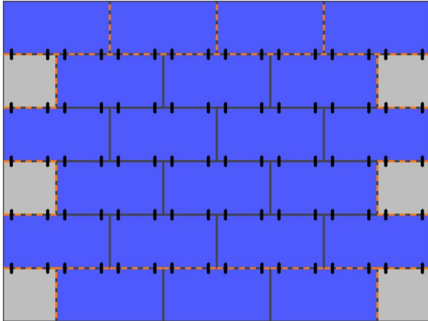
Abb.: Verlegung 1,0x0,5m große Platten in Kombination mit 0,5x0,5m großen Platten. Steckverbinder schwarz dargestellt, Klebelinien rot dargestellt.
