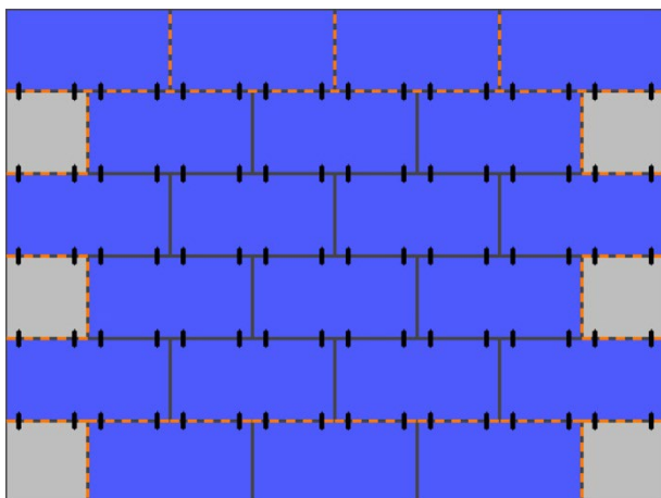
Abb.: Verlegung 1,0x0,5m große Platten in Kombination mit 0,5x0,5m (geschnitten aus 100x50cm Platten) großen Platten. Steckverbinder schwarz dargestellt, Klebelinien rot dargestellt.
