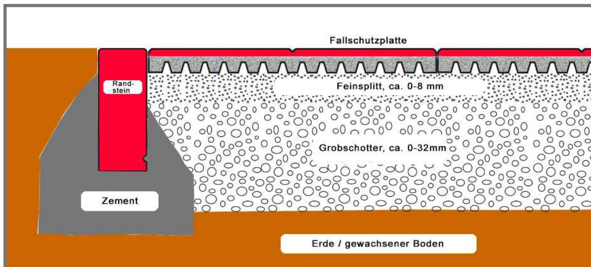
Bsp.: Fallschutzplatte, ca. 1x1m, verlegt auf Schotteruntergrund, fixiert durch Seitenverklebung.
