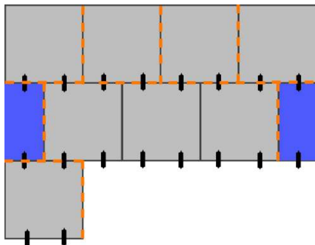
Abb.: Verlegung von 0,5x0,5m großen Platten in Kombination mit 0,25x0,5m großen Platten.
